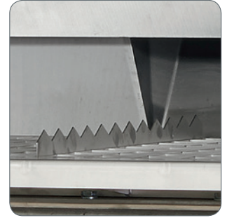
Zick-Zack Messer zum rationellen Öffnen der Säcke
